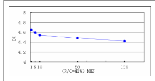
Dielectric constant 介电常数
